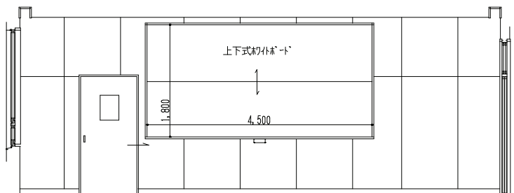
[設置例]アルミ枠上下式ホワイトボード（ホーローホワイト） 4500×1800
